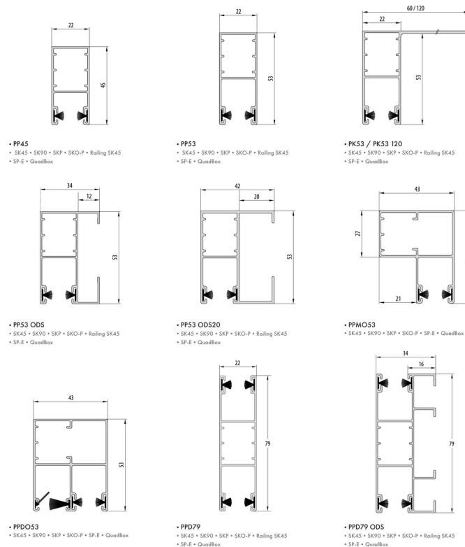
Auswahl gängiger Führungsschienen-Querschnitte für Vorbau- und Unterputzrollläden (Maße in mm)
